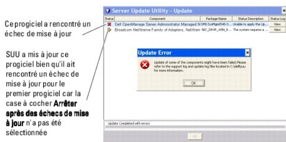
Figure 2-16. Continuation après une erreur de mise à jour
