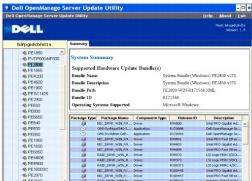
Figure 2-19. Détails au niveau d'un lot
