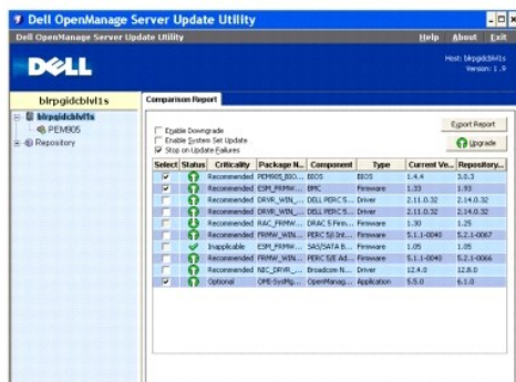
Figure 2-13. Option Arrêter après des échecs de mise à jour sélectionnée
